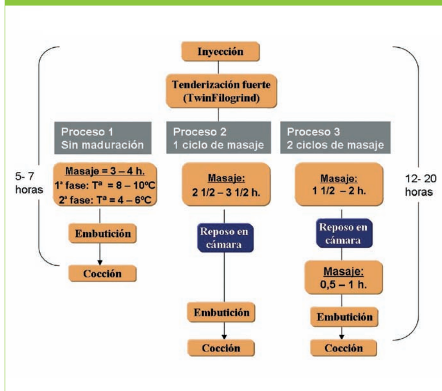
Figura 1. Posibilidad de procesos con una línea Metalquimia
