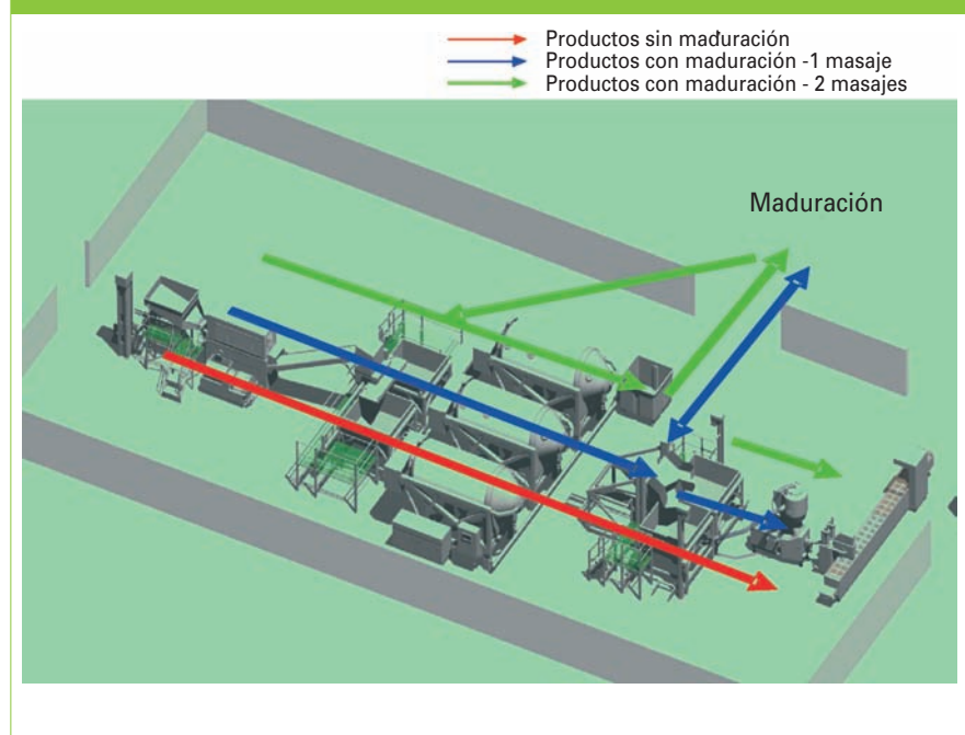
Figura 2. Diseño tradicional y lay-out de una planta
