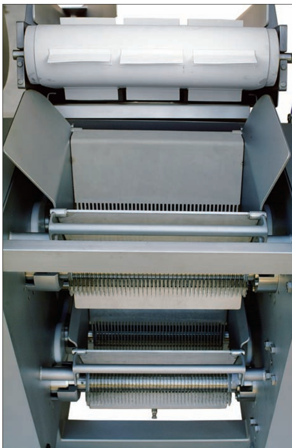
Foto 1. Tenderizadora Twinfilgrind de doble acción.
